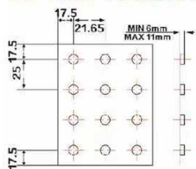
3 \Phi 12*35*35 直片 波纹片 (边缘波纹)
