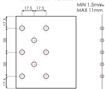
7 \Phi 7*35*35 直片 波纹片 (边缘波纹)
