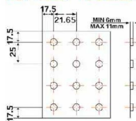
4 \Phi 9.52*35*35 直片 波纹片 (边缘波纹)
